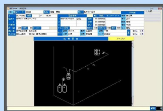
配管図面
